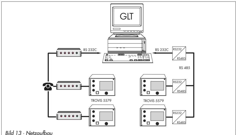
Bild 13 · Netzaufbau
