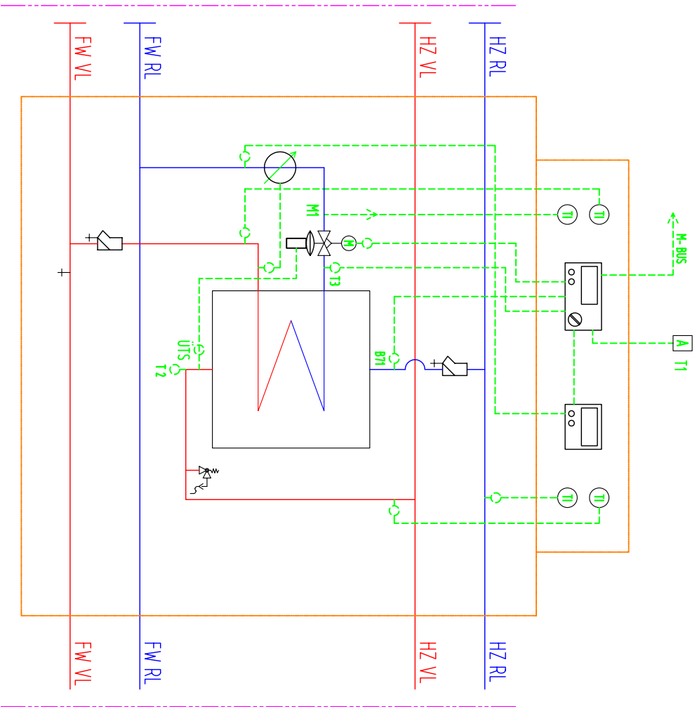
UTS omnit mechanischen Thermostat 125 - 175 kW
